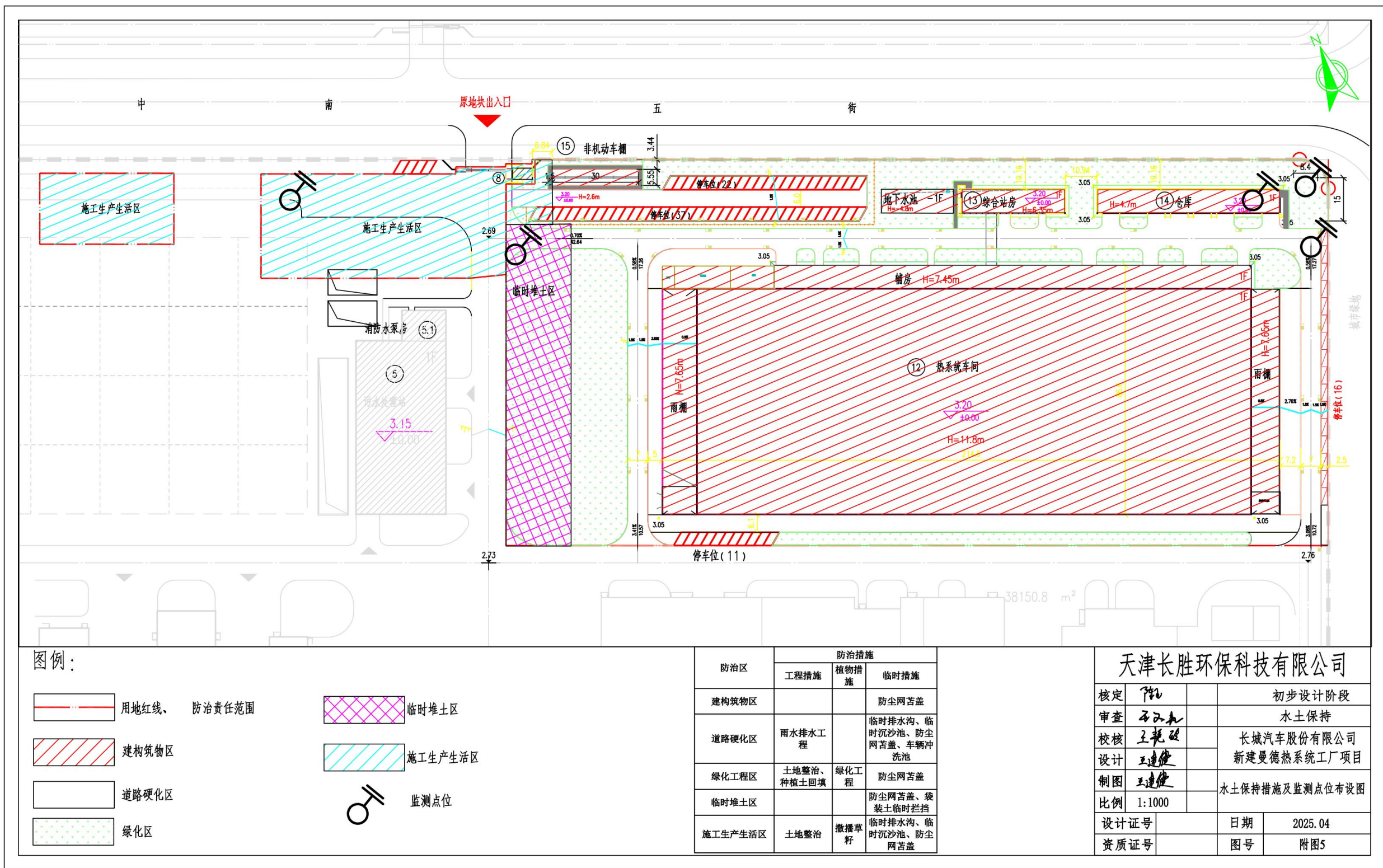
附图 5 水土保持措施及监测点位布设图
