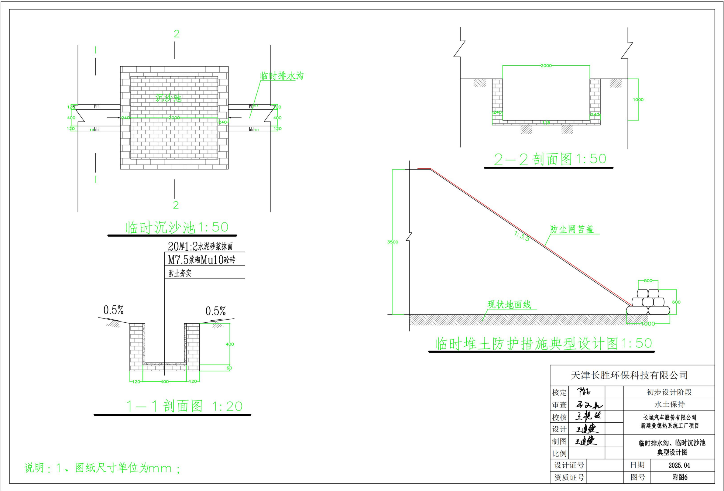
附图 6-2 临时排水沟、临时沉沙池典型设计图
