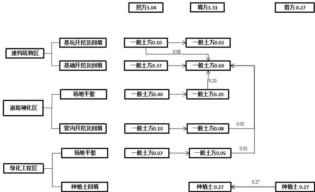
图 2-4 土石方平衡及流向框图（图中单位：万 \text{m}^3 ）
