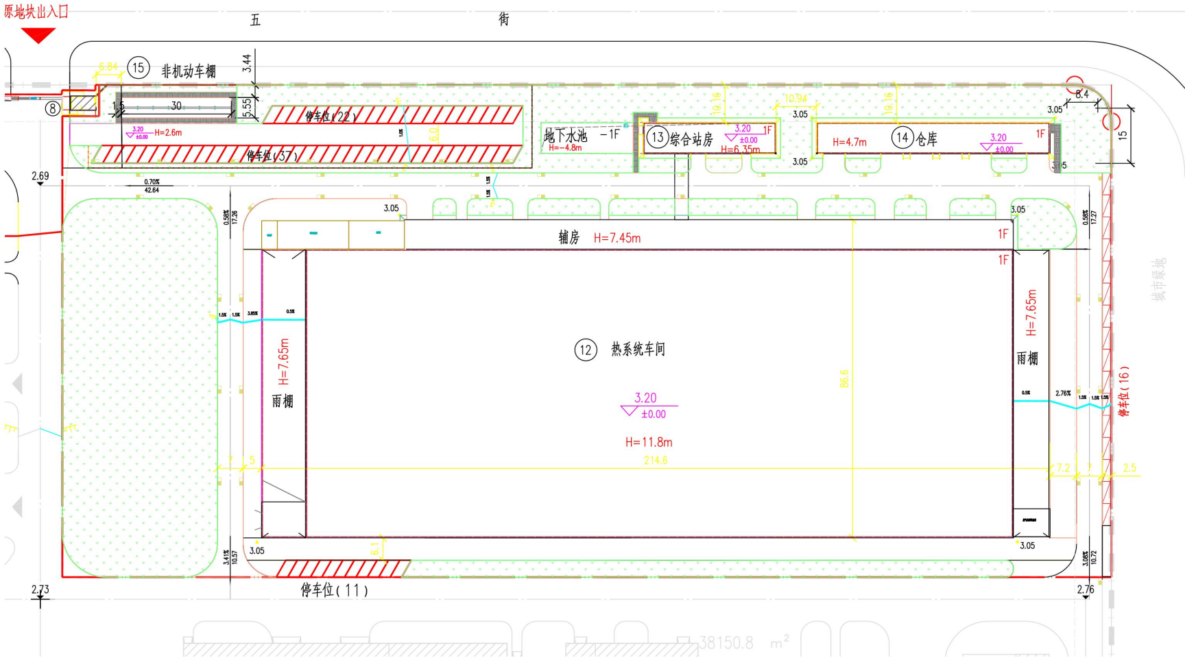
图 2-2 项目总平面布置图
